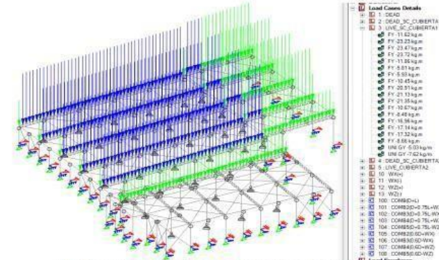
Figura 11. Modelo matemático tridimensional/ Carga viva en cuerpo 2, CV1=40 kg/m 2 .
